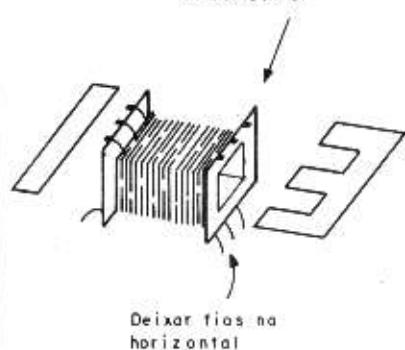
Montagem das chapas E e I no carretel
