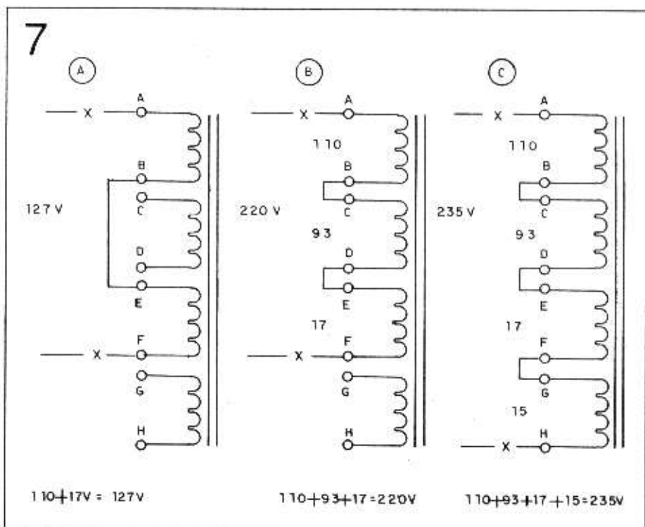
Associação em série de enrolamentos primários
