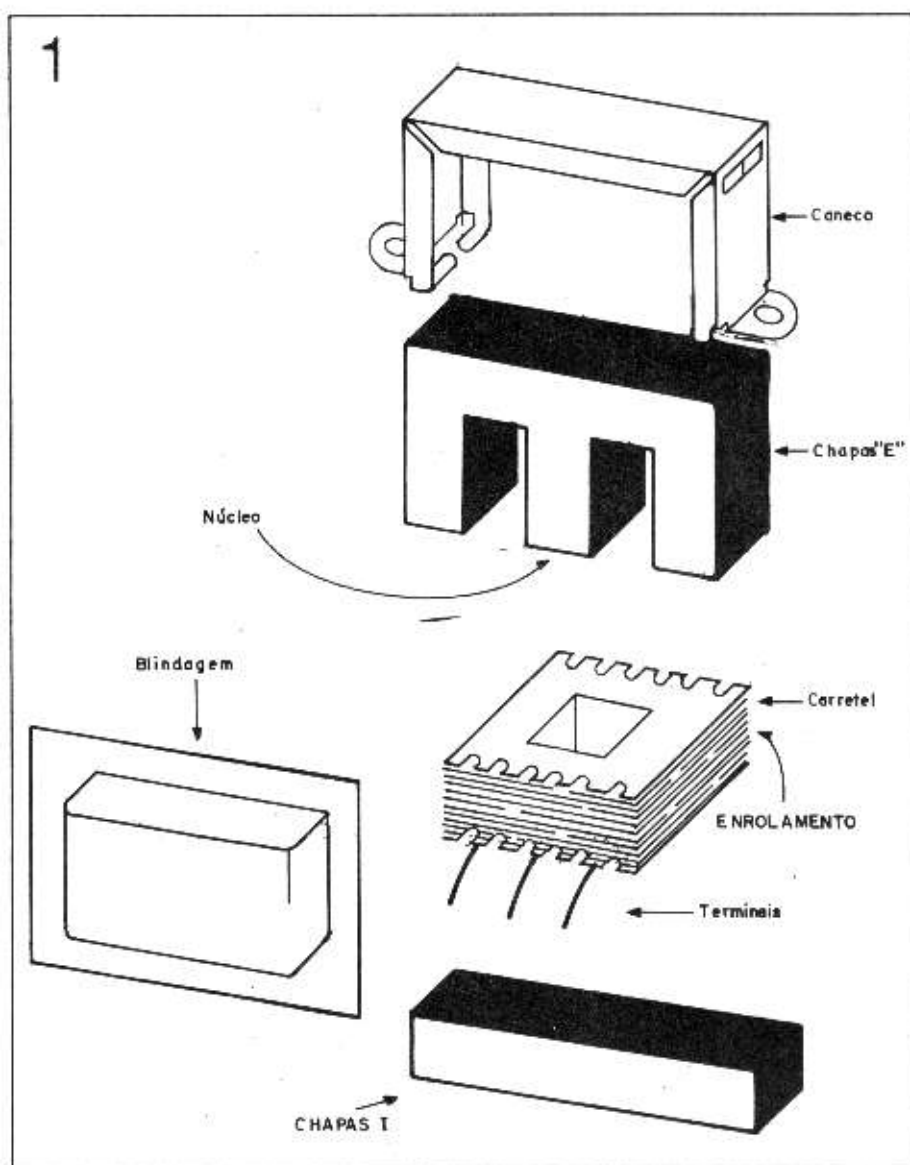
Vista explodida de um transformador comum
