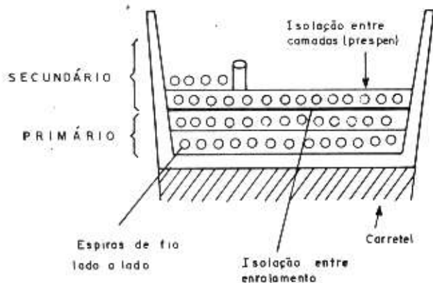
Corte de um carretel mostrando o aspecto do enrolamento em andamento
