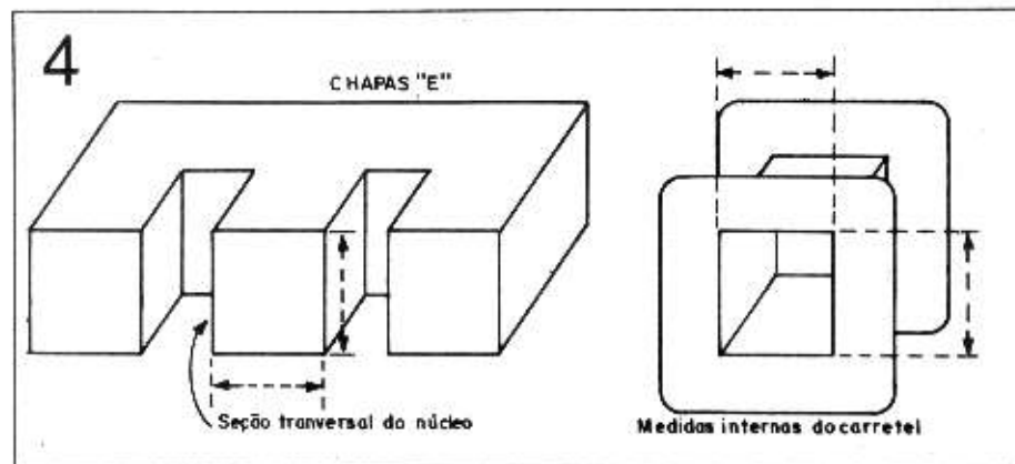
Núcleo e carretel
