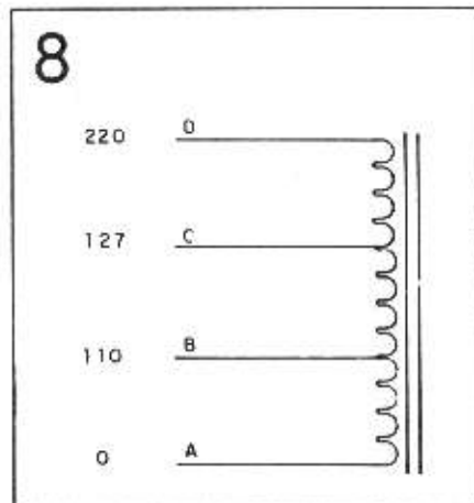
Enrolamento primário com derivação
